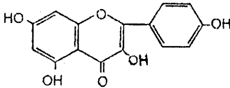
Kaempferol
