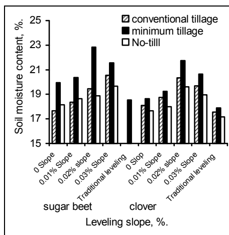
b. Moisture content.
