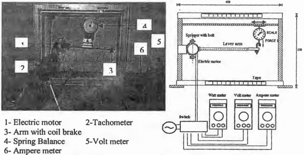
Fig. 2: Indicate the Prony brake apparatus
