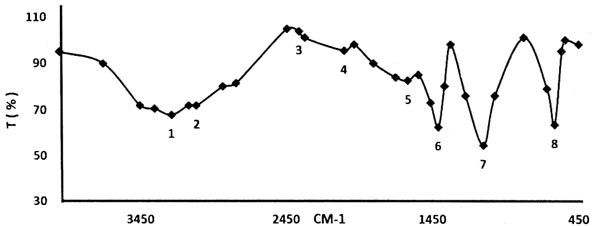
Fig. 5. IR of orange peels
