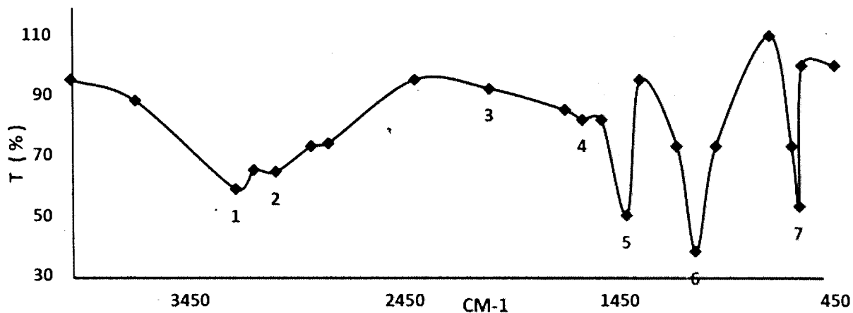
Fig. 4. IR of lemon peels
